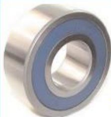
1030224PFI BALERO ALTERNADOR CHRYSLER NIPPONDENSO(336) ANTES B3360 15 X 32 X 11
